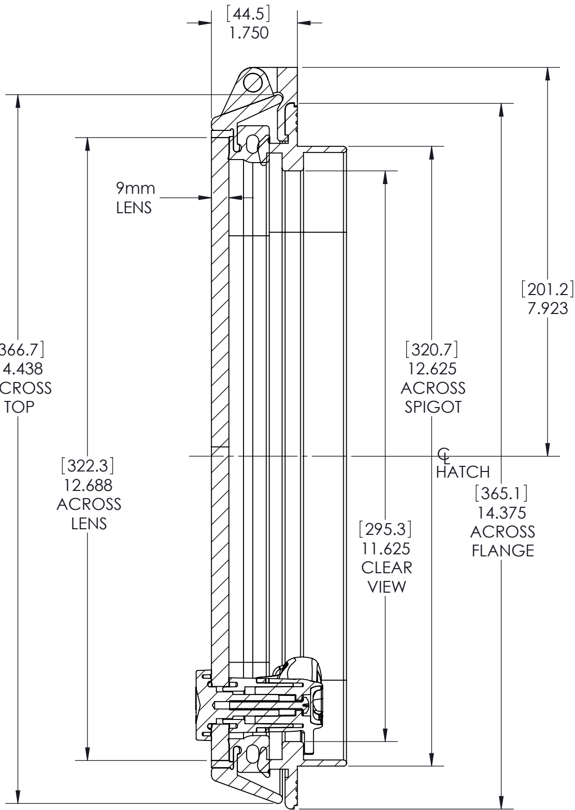
SECTION A-A
